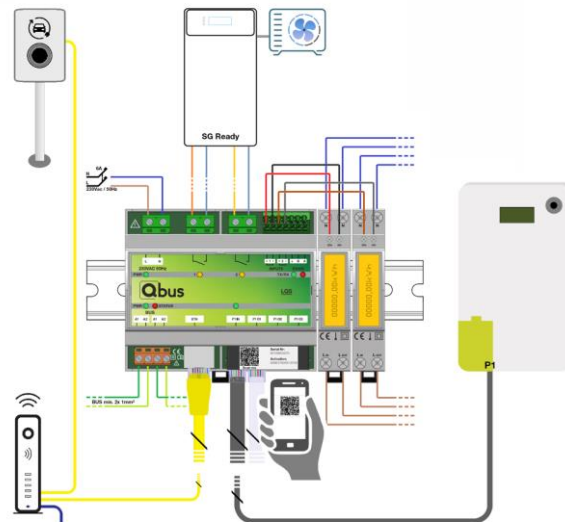
Figuur 3 Aansluitschemavoorbeeld
