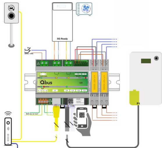
Figure 3 Exemple de schéma de raccordement
